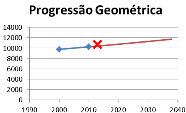
Gráfico 15: Projeção populacional com Modelo Geométrico
