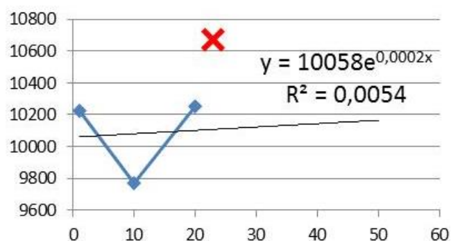
Gráfico 18: Projeção Populacional com Modelo Exponencial
