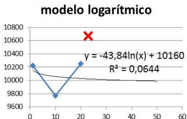
Gráfico 19: Projeção populacional com Modelo Logarítmico
