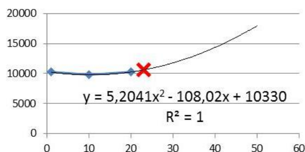
Gráfico 20: Projeção populacional com Modelo Polinomial de Segunda Ordem
