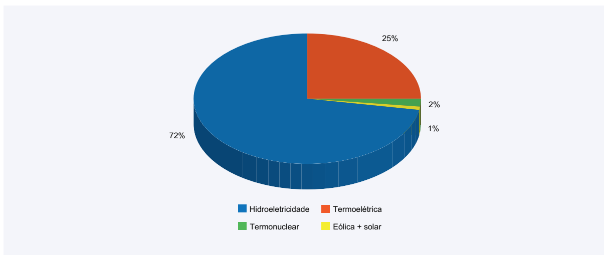
Figura 24 – Situação da matriz elétrica nacional em dezembro de 2010 21
