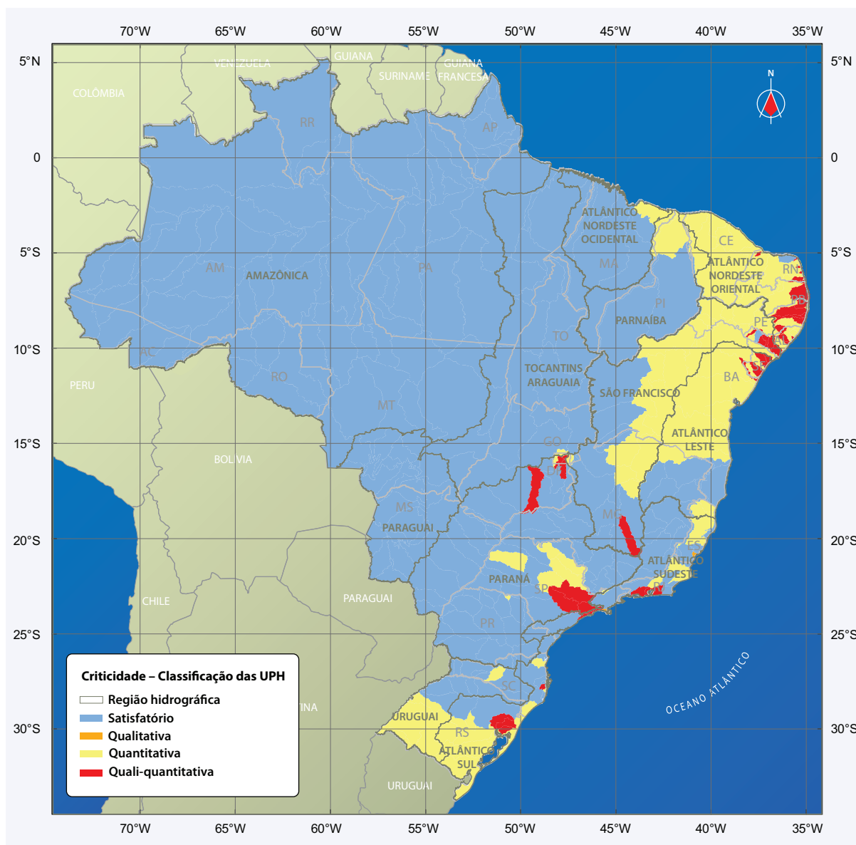
Figura 31 – Balanço quali-quantitativo nas Unidades de Planejamento Hídrico (UPH) brasileiras
