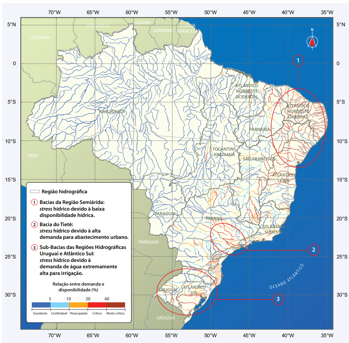
Figura 26 – Situação dos principais rios brasileiros quanto à relação demanda versus disponibilidade hídrica superficial 26
