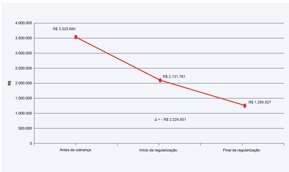
Figura 47 – Variação do valor total da cobrança antes (projeção) e depois do processo de regularização na Bacia do Rio São Francisco, nos perímetros irrigados da Companhia de Desenvolvimento dos Vales do São Francisco e do Parnaíba (Codevasf)
