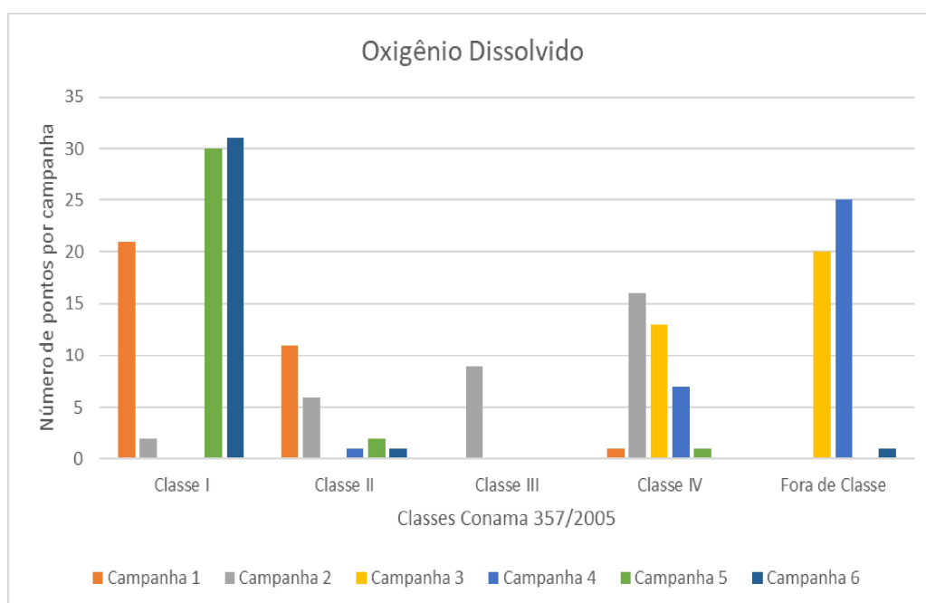
Figura 7.4. Resultados acumulados para o parmetro de Oxigênio Dissolvido.
