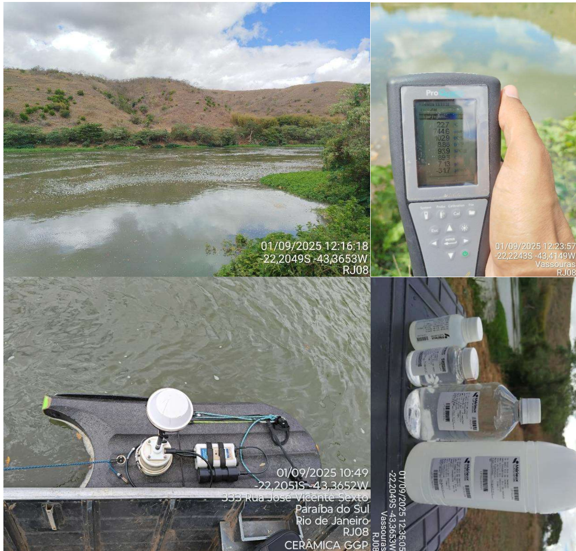
Figura 4.16. Registros fotográficos do ponto RJ08 - Cerâmica GGP, destacando a seção de medição, a medição de vazão e de parâmetros de qualidade da água, e a coleta de amostras de água.
