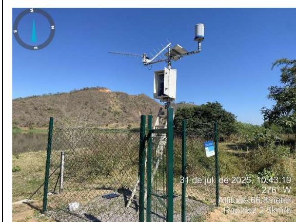
Figura 2.3 - Vista externa da PCD.
