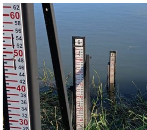
Figura 2.2 Nível marcado na régua.
