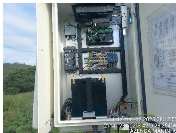
Figura 2.6 Vista interna da PCD.
