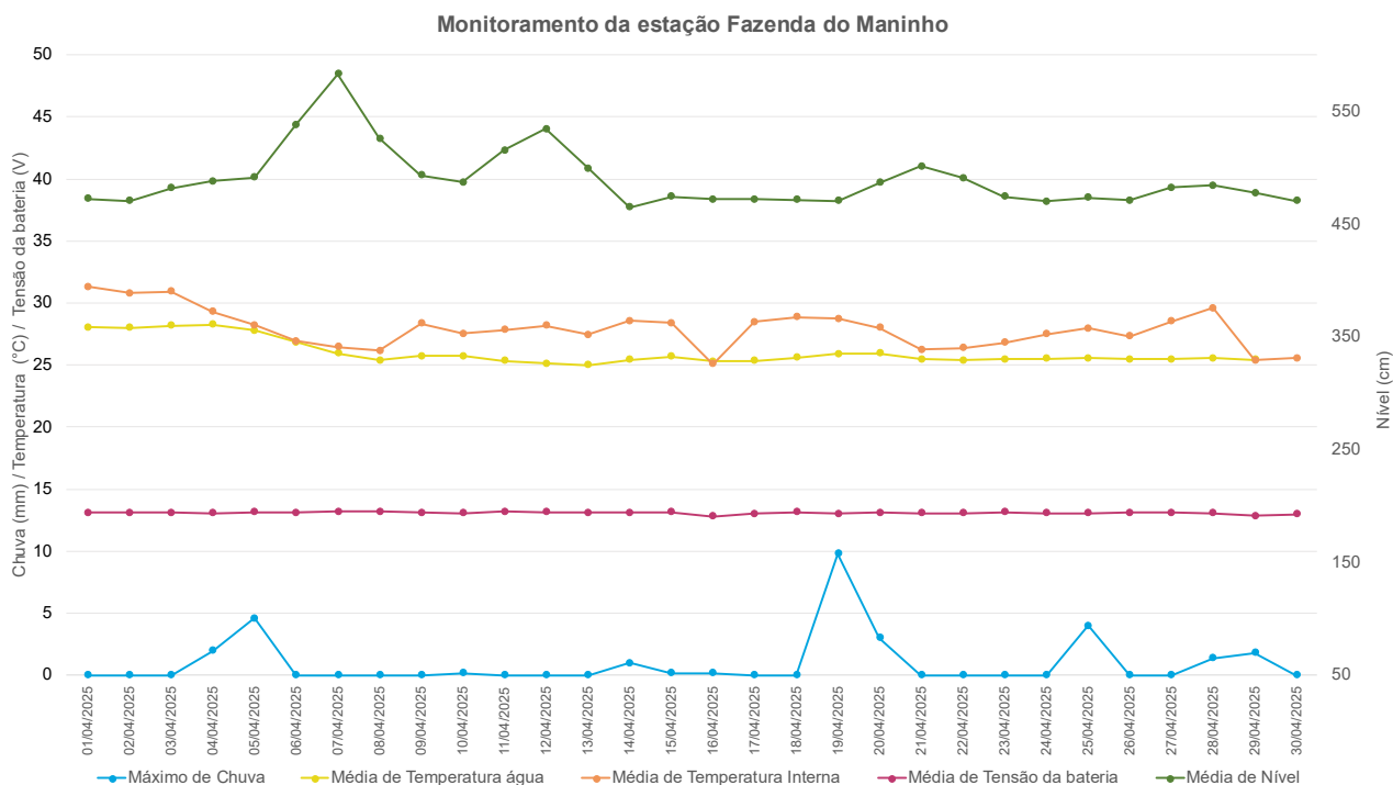
Figura 2.15 Parâmetros monitorados na estação.
